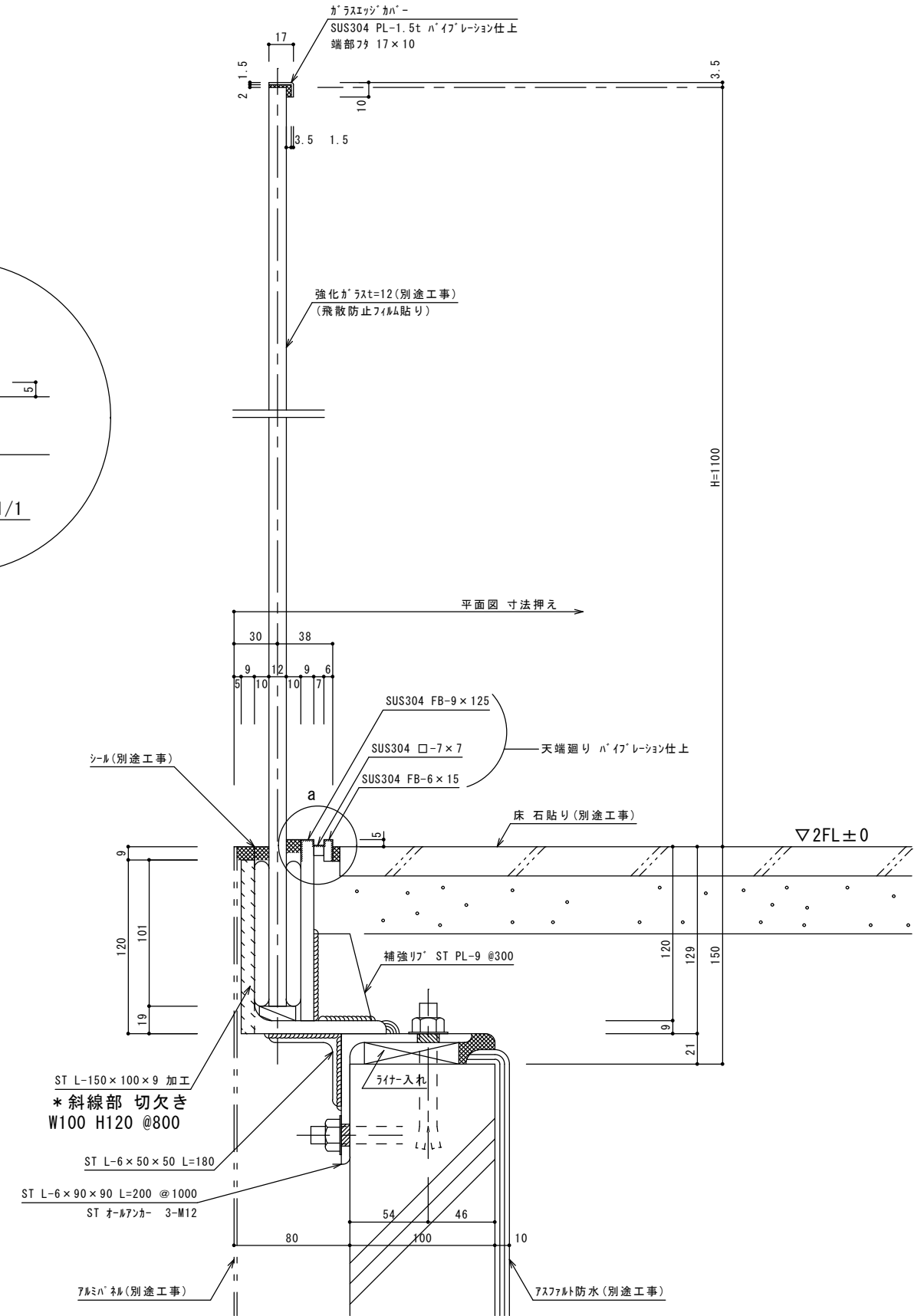
断面詳細図 S=1/2
