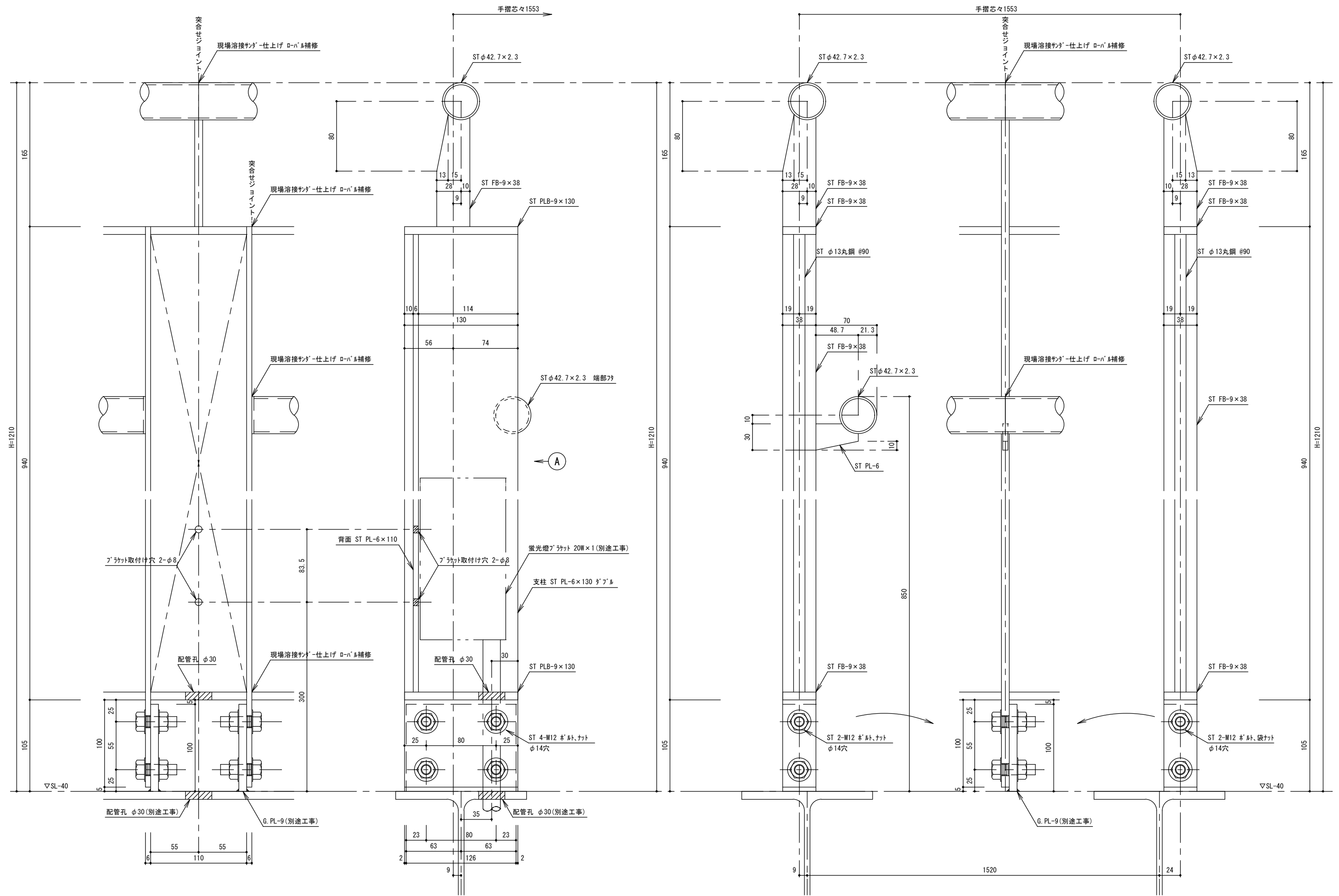
A 立面詳細 S=1/2
