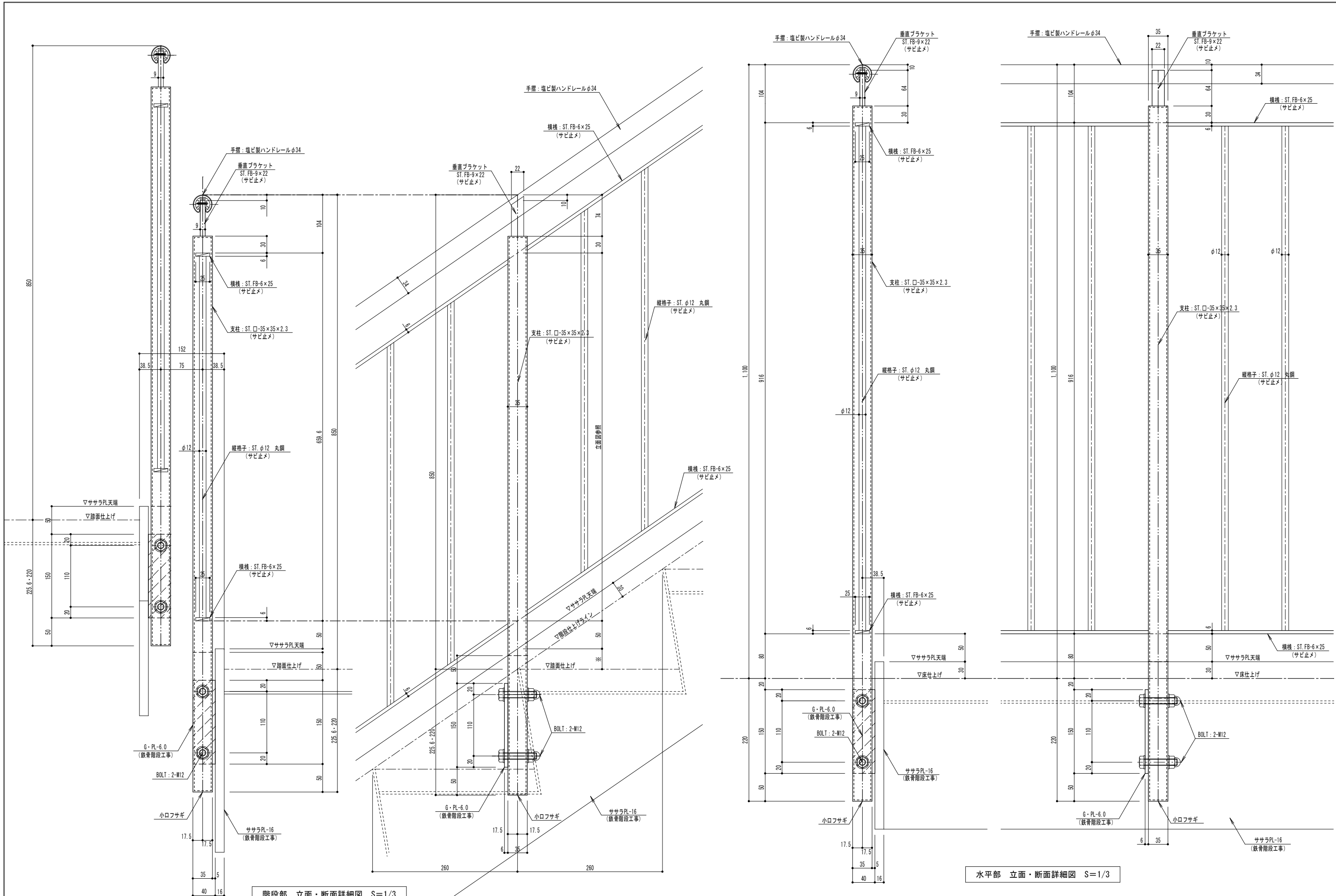
階段部 立面・断面詳細図 S=1/3
